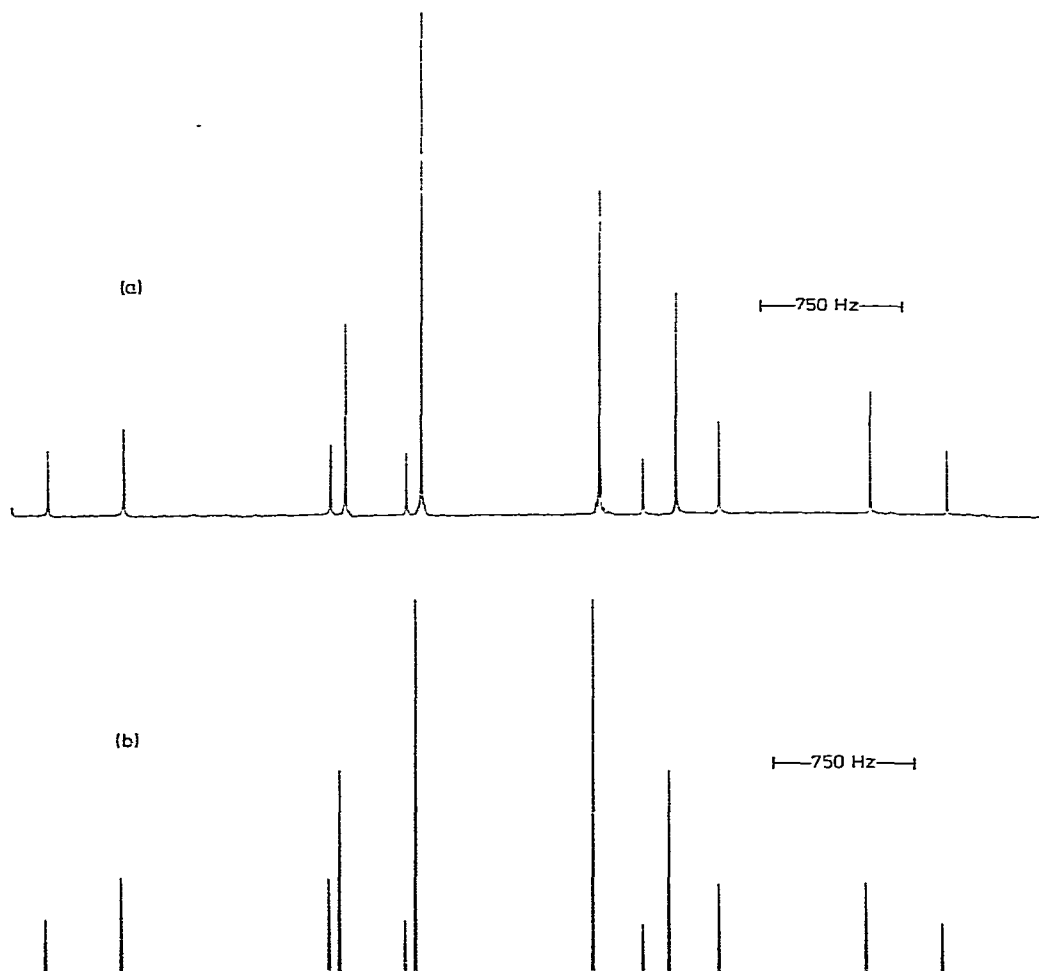
Fig. 2. ^{31}\text{P}\{^1\text{H}\} -NMR-Spektrum (in Toluol, ext. Standard 85 proz. Phosphorsäure/ \text{D}_2\text{O} ) von [\text{Cl}(\text{CH}_2)_3(\text{H}_{11}\text{C}_6)_2\text{P}](\text{Cl})\text{PtP}(\text{C}_6\text{H}_{11})_2\text{CH}_2\text{CH}_2\text{CH}_2 [(a) gemessen, (b) computer-simuliert].
